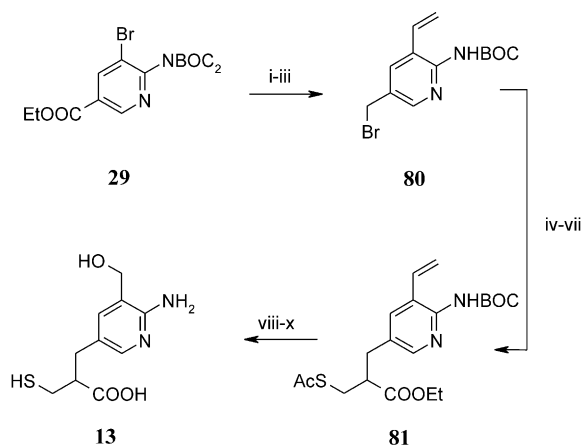
Scheme 9. Conditions: (i) Bu 3 SnCHCH 2 , (Ph 3 P) 4 Pd, 1,2-dichloroethane; (ii) DIBAL, THF; (iii) Ph 3 P, CBr 4 , CHCl 3 ; (iv) (EtOCO) 2 CH 2 , NaH, DMF; (v) KOH, EtOH/CH 2 Cl 2 ; (vi) Et 2 NH, CH 2 O (aq) , CH 2 Cl 2 ; (vii) Et 3 N, AcSH; (viii) O 3 , EtOH, then NaBH 4 , water; (ix) Ac 2 O, KHCO 3 ; (x) HCl (aq) .
